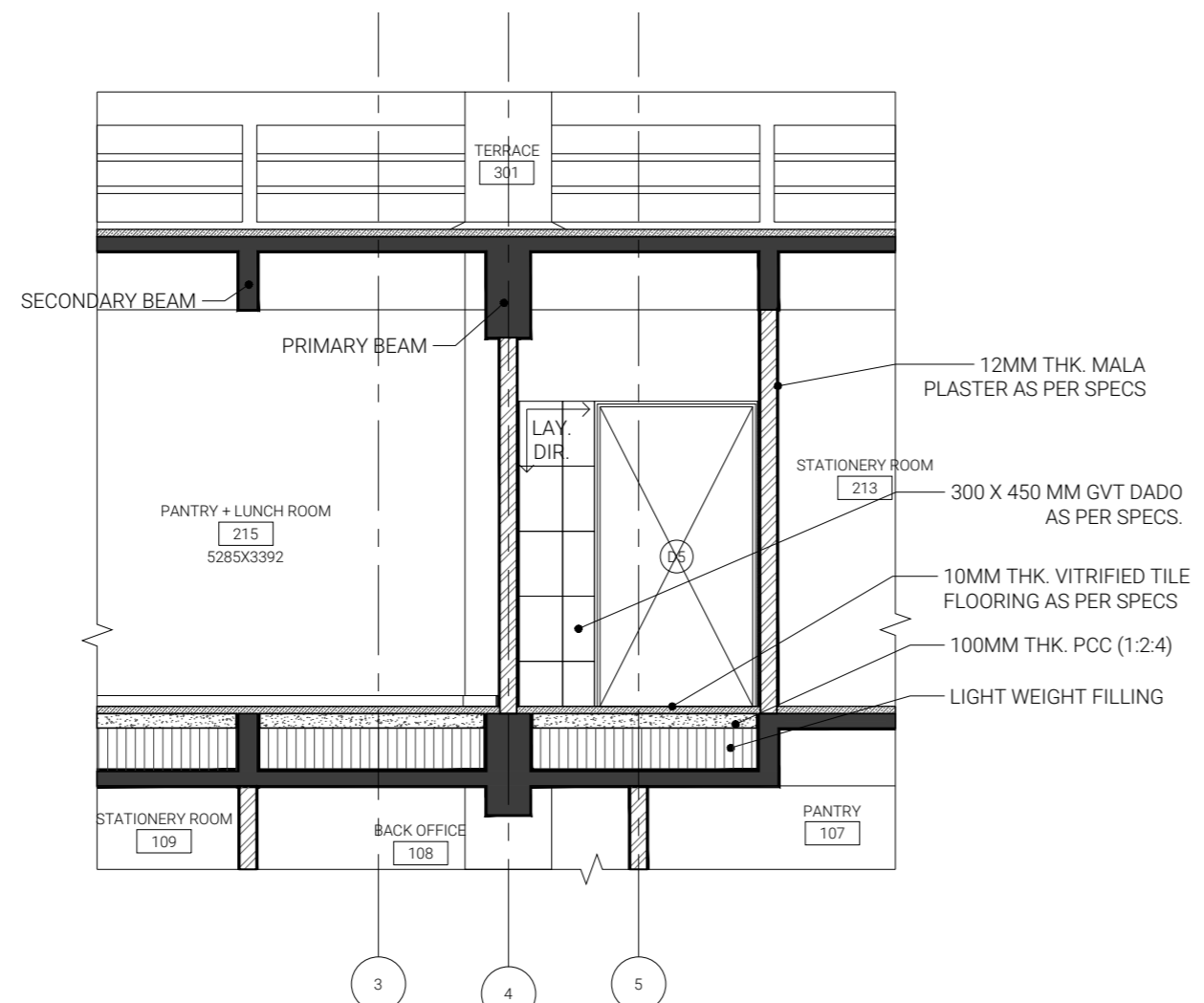
4 ELEVATION 3 1:50
