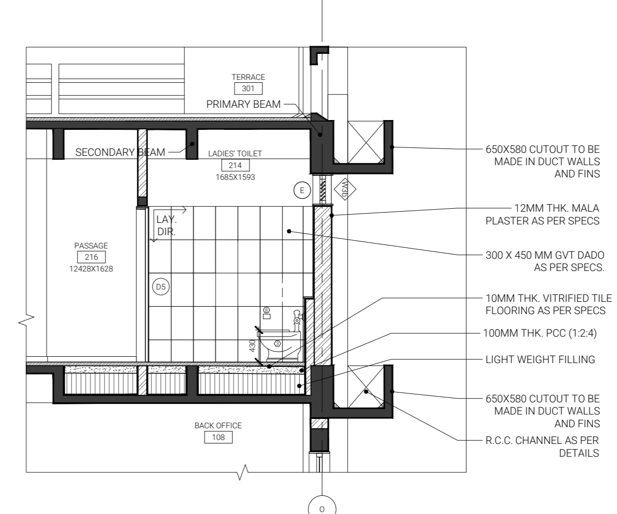
5 ELEVATION 4 1:50
